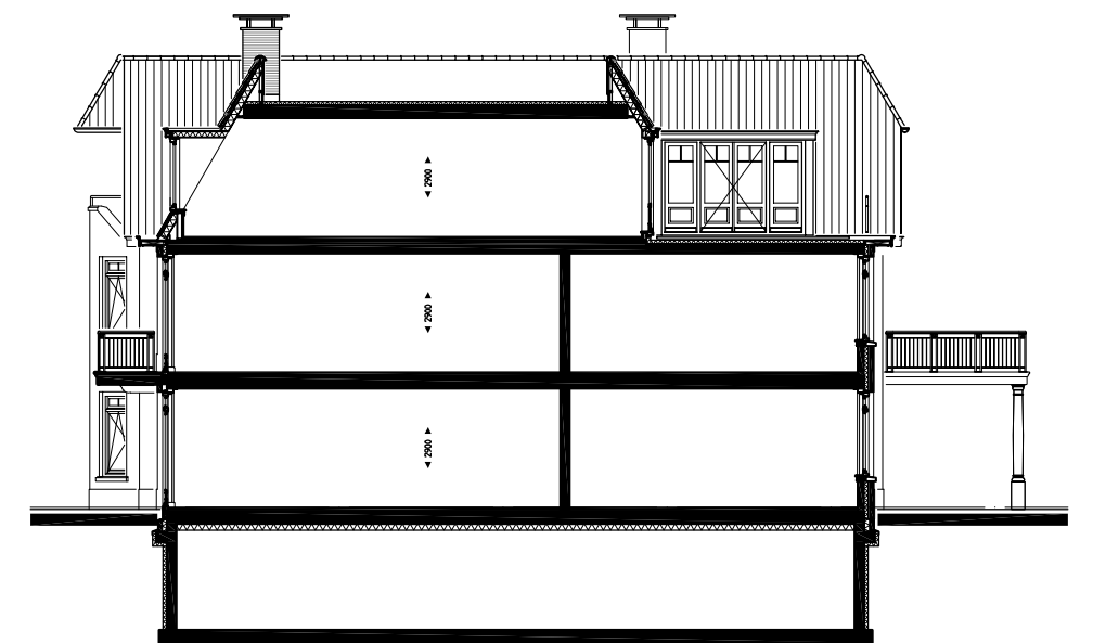
Doorsnede A-A
