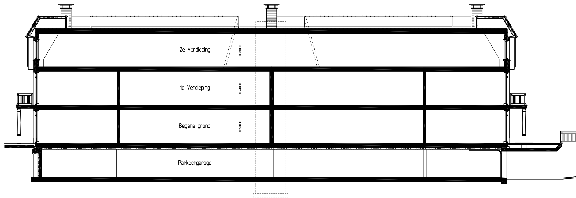
Doorsnede B-B
